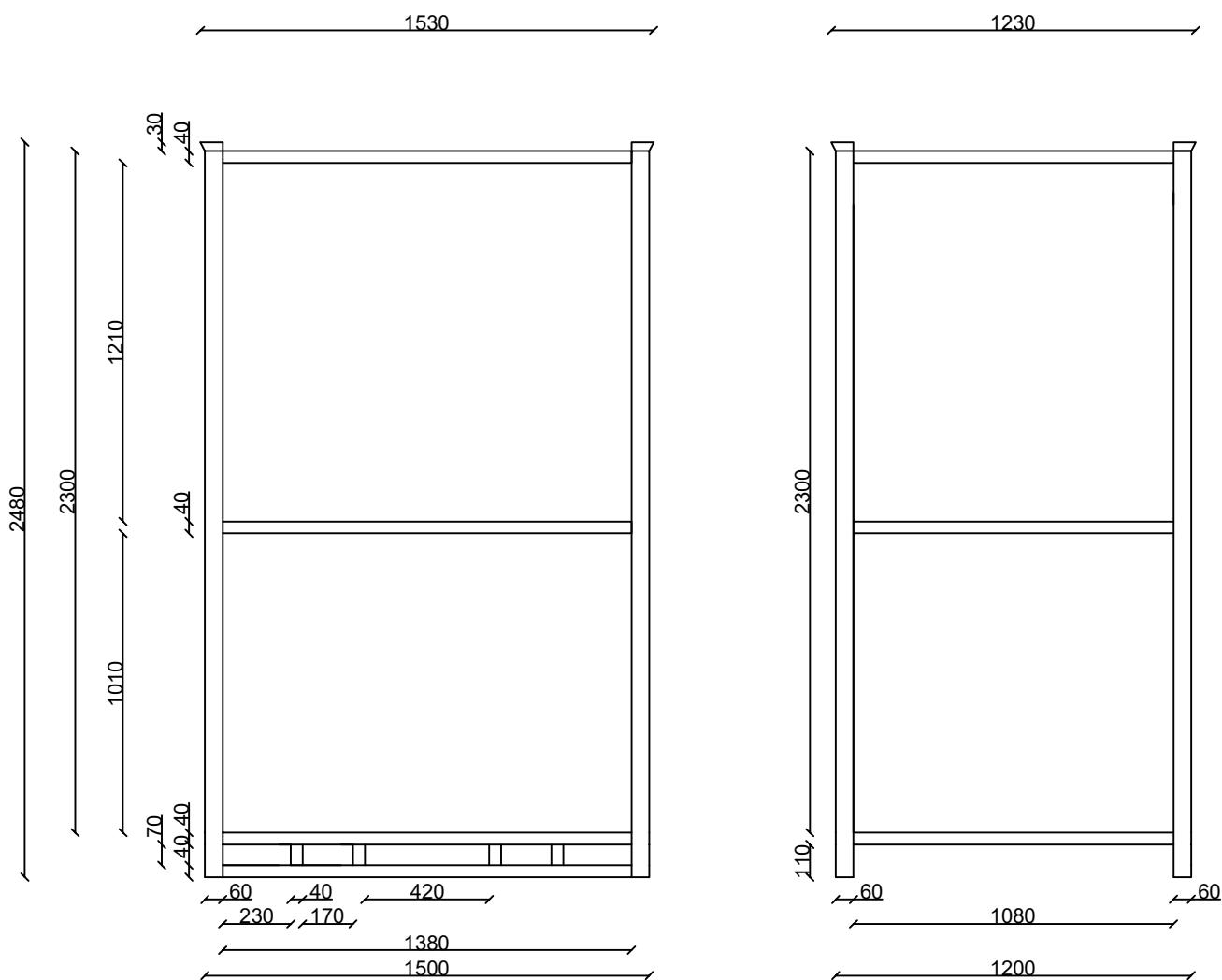
MP054-28 PEDANE PALLET CON SPONDE
