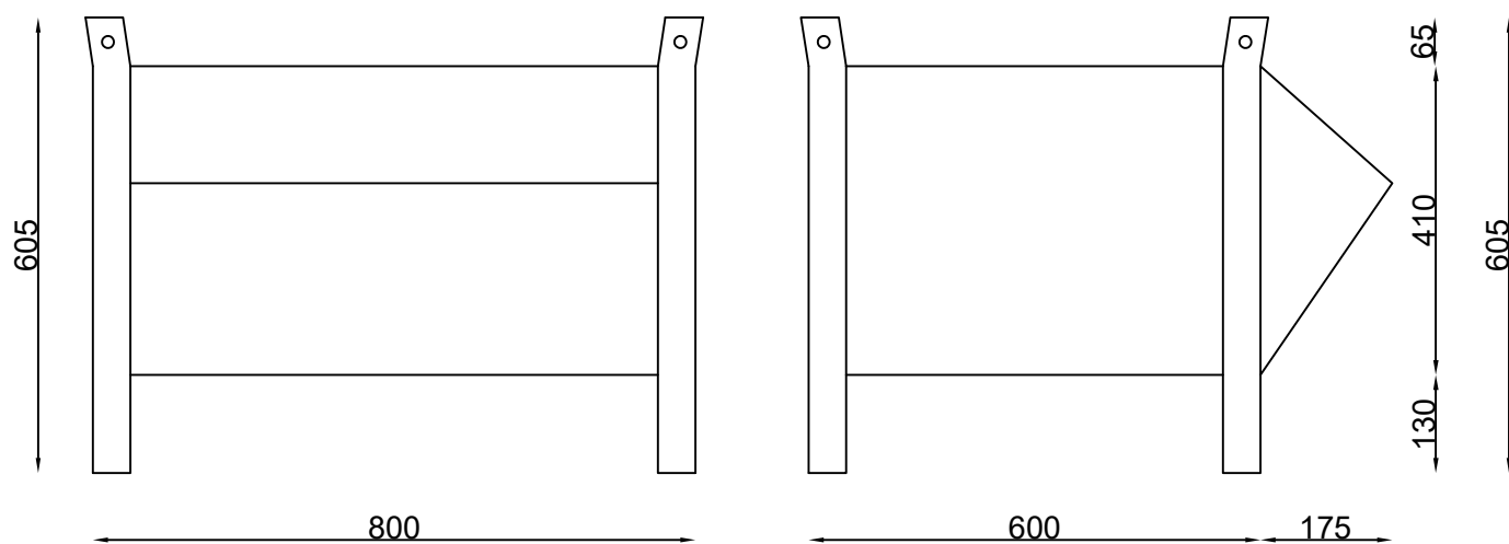
MC037-32: Contenitore in lamiera a BOCCA di LUPO tara kg.35
